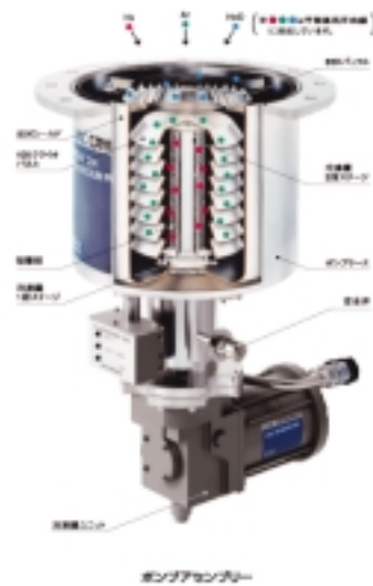
クライオポンプのしくみ
