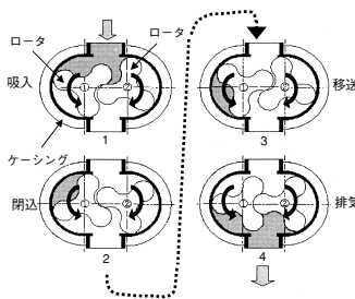
多段ルーツ型
