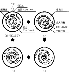
スクロール型
