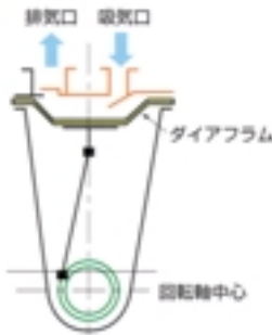
ダイアフラム型
