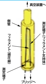
ピラニ真空計の構造
