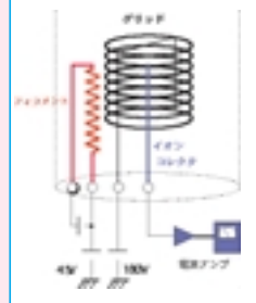
B-A真空計の構造
